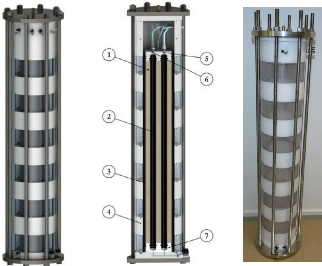
Abb. 1: Systemtriaxialzelle zur Bestimmung der hydraulischen Systemdichtheit von Erdwärmesonden. Links: isometrische Darstellung. Mitte: Schnittdarstellung mit Verfüllmaterial (1), Sondenrohren (2), Latexmembran (3), Druckbehälterwand (4) bestehend aus abwechselnd gestapelten transparenten und opaken Ringen, Fluidkreiseintritt (5), Fluidkreisaustritt (6) am oberen Probenstempel und unterem Probenstempel (7). Rechts: Systemtriaxialzelle im aufgebauten Zustand.
