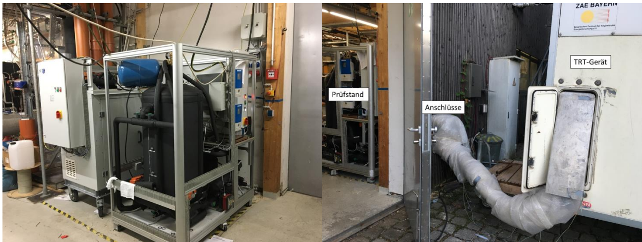
Abb. 2: links: Fertig aufgebauter Prüfstand; rechts: TRT-Gerät an künstlicher Erdwärmesonde angeschlossen.
